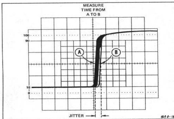
Fig. 14. Pulse jitter.
