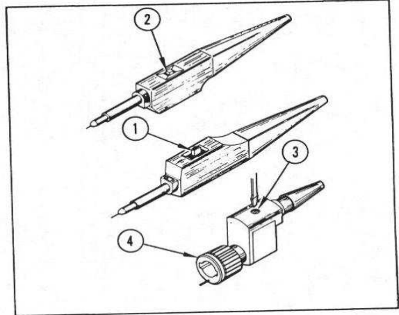
Fig. 2. P6062A probe.
