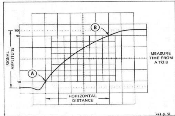
Fig. 8. Risetime.
